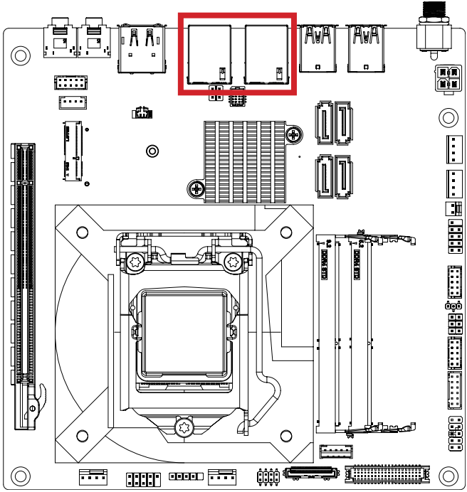
LAN Connector
